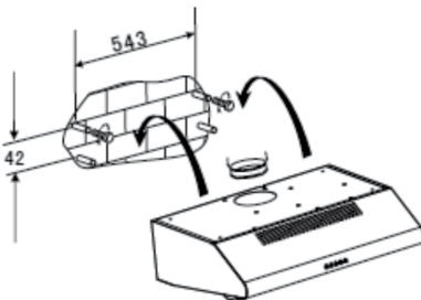
60cm hood
